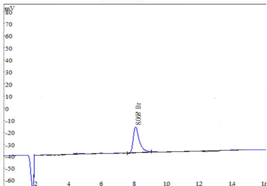
固定発生源から排出される気体中の 臭化水素 の測定 HJ544-2016
