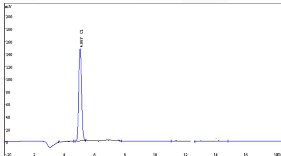
固定発生源から排出される気体中の 塩化水素 の測定 HJ549-2016
