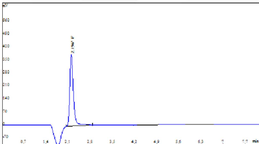
固定発生源から排出される気体中の フッ化水素 の測定 HJ688-2019
